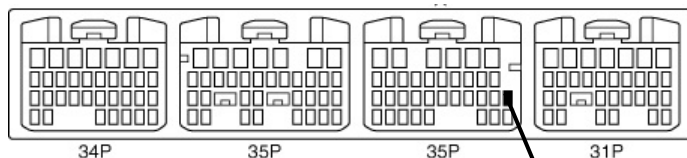
①ECUコネクタ35P
