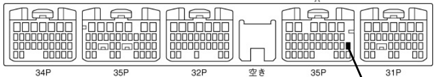
①ECUコネクタ35P
