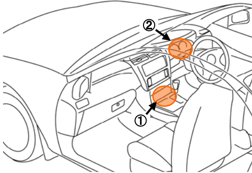
①中継コネクタ26P(白)
