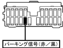
②メーターユニットコネクタ22P(緑)
