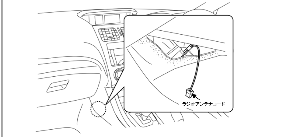
車両側ラジオアンテナコードの位置
