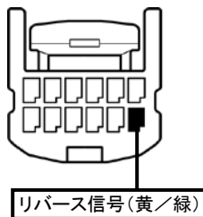
②バックランプコネクタ12P(白)
