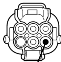
②バックランプコネクタ6P(灰)
