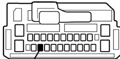
オーディオコネクタ24P(灰)
