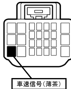
③メーターユニットコネクタ32P(灰)
