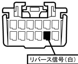
②ヒューズボックス内コネクタ12P(緑)
