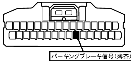
③メーターユニットコネクタ32P(灰)
