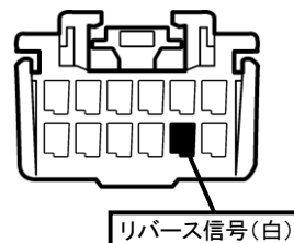
③ヒューズボックス内コネクタ12P(緑)
