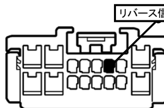
①ヒューズボックス内コネクタ16P(緑)
