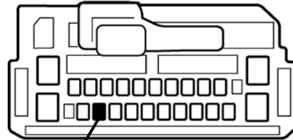
車速信号(青)
