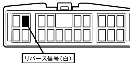
②ヒューズボックス内コネクタ20P(白)
