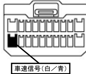
①オーディオコネクタ20P(白)
