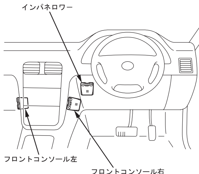
インパネ付近への取り付け例
