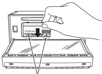
下部ツメ
