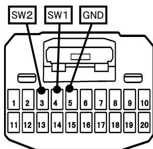
車両ハーネス20Pコネクタ(白)
