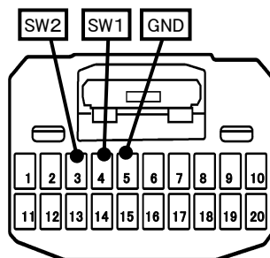
車両ハーネス20Pコネクタ(白)
