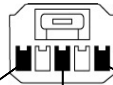
オプションコネクタ5P(白)
