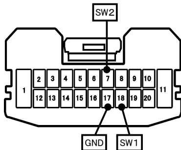
車両ハーネス20Pコネクタ(白)
