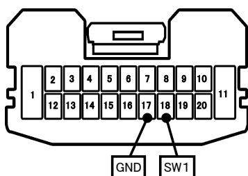
車両ハーネス20Pコネクタ(白)
