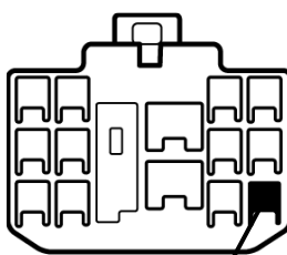
②中継コネクタ14P(白)
