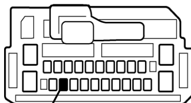
オーディオコネクタ24P(灰)
