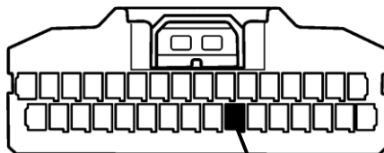
パーキングブレーキ信号(橙)
