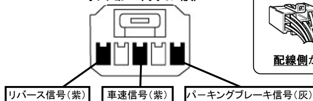
オプションコネクタ5P(灰)
