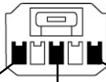
オプションコネクタ5P(灰または白)
