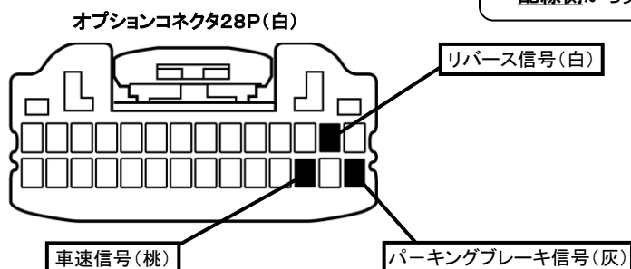
配線側から見た図
