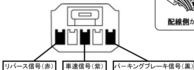
オプションコネクタ5P(灰)
