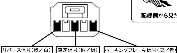
オプションコネクタ5P(白)
