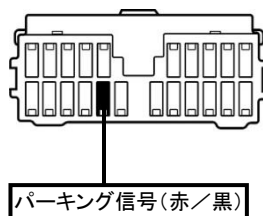
②メーターユニットコネクタ22P(緑)
