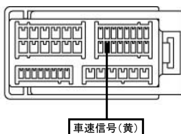
①中継コネクタ42P(白)
