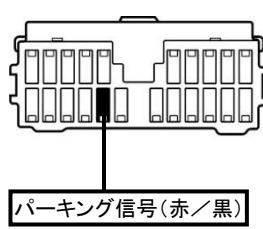
②メーターユニットコネクタ22P(緑)
