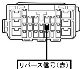
①中継コネクタ26P(白)
