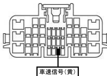
①中継コネクタ38P(白)
