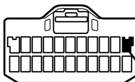
②ヒューズボックス右側22Pコネクタ(青)
