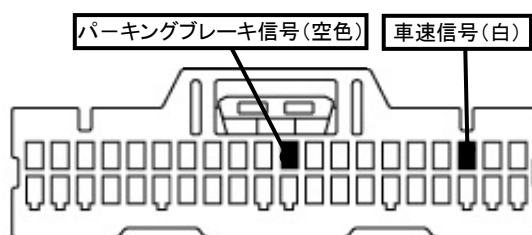
①メーターユニットコネクタ40P(白)
