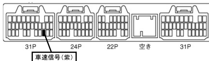
①ECUコネクタ31P
