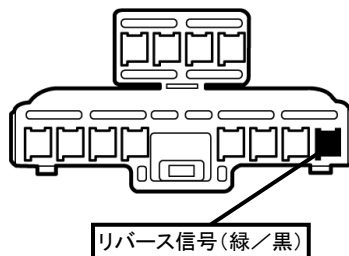
②ヒューズボックス内コネクタ4P+8P(緑)
