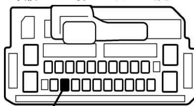
変換ハーネス側のコネクタ24P(灰)
