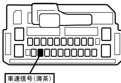
オーディオコネクタ24P(灰)
