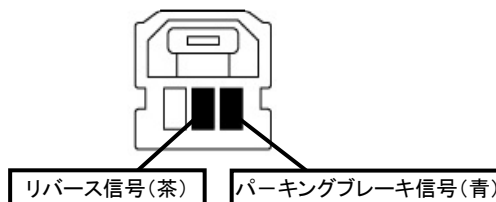
変換ハーネス側のコネクタ3P(灰)
