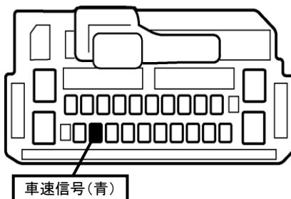
変換ハーネス側のコネクタ24P(灰)
