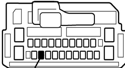
車速信号(橙)
