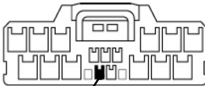
車速信号(青)
