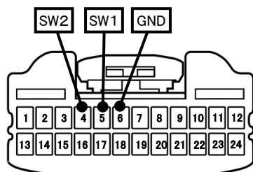
24Pコネクタ(白)
