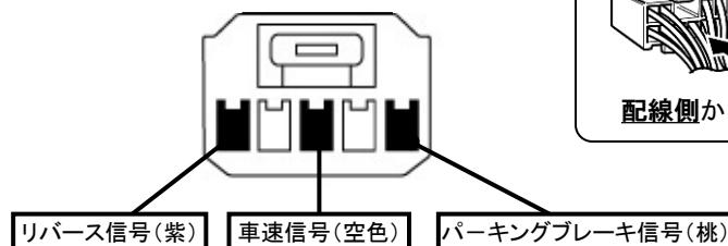
車両ハーネス5Pコネクタ(灰)
