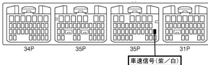
①ECU35Pコネクタ
