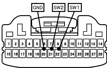
車両ハーネス28Pコネクタ(白)
