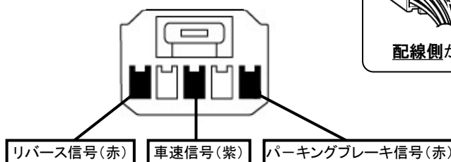
オプション5Pコネクタ(白)
