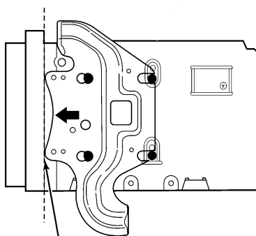
ブラケットの端をこの面に当てる
