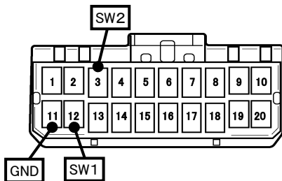
車両ハーネス20Pコネクタ(青)
