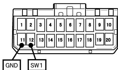
車両ハーネス20Pコネクタ(青)
