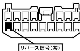
②ヒューズボックス内コネクタ16P(白)
