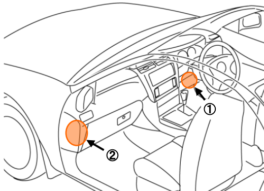
①パワーステアリングコントロールユニットコネクタ10P
