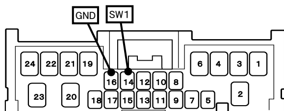
車両ハーネス24Pコネクタ(白)
