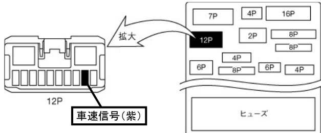
ヒューズボックス内コネクタ12P(緑)
