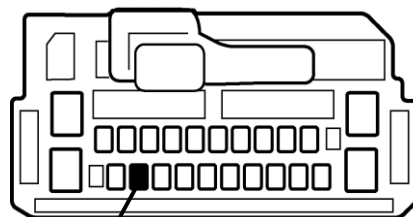
車速信号(紫)
