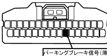
③メーターユニットコネクタ32P(灰)
