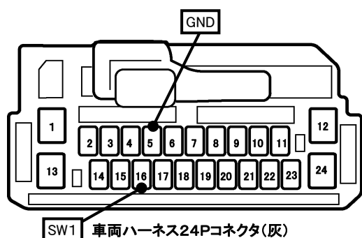
SW1 車両ハーネス24Pコネクタ(灰)
